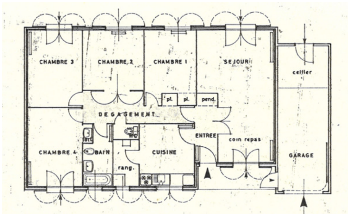
Plan d'un pavillon type V © Fonds Paul Bouron
